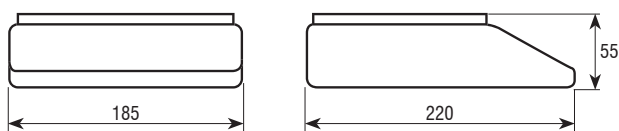
Dimensões (mm)
